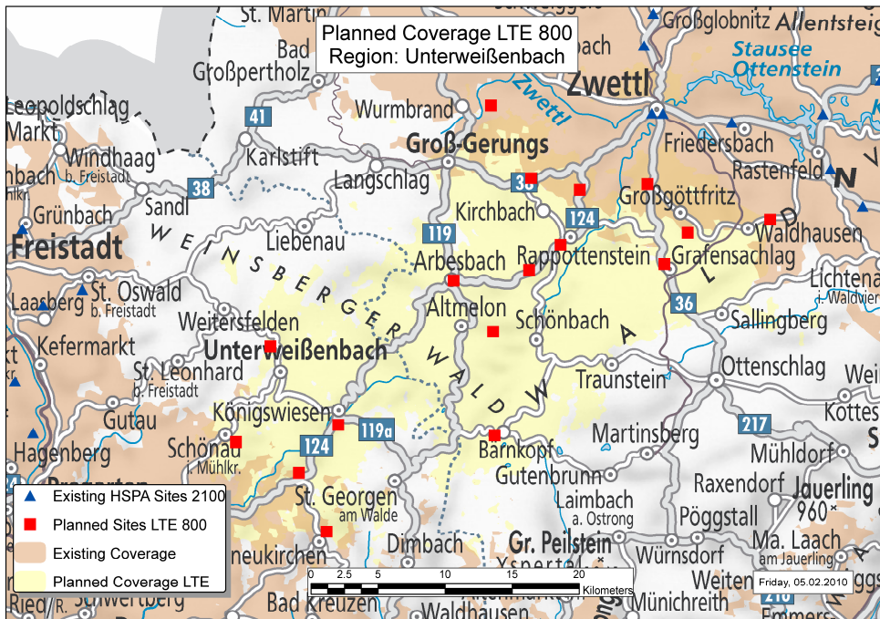
Abbildung 30: LTE-Referenzszenario Unterweißbach Quelle: Brancheninformation 2/2010
