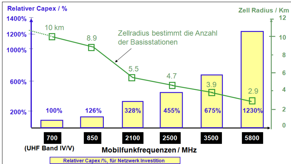
Abbildung 12: Die Frequenz bestimmt die Reichweite – und damit die Kosten Quelle: Forge/Blackman/Bohlin 2007.
