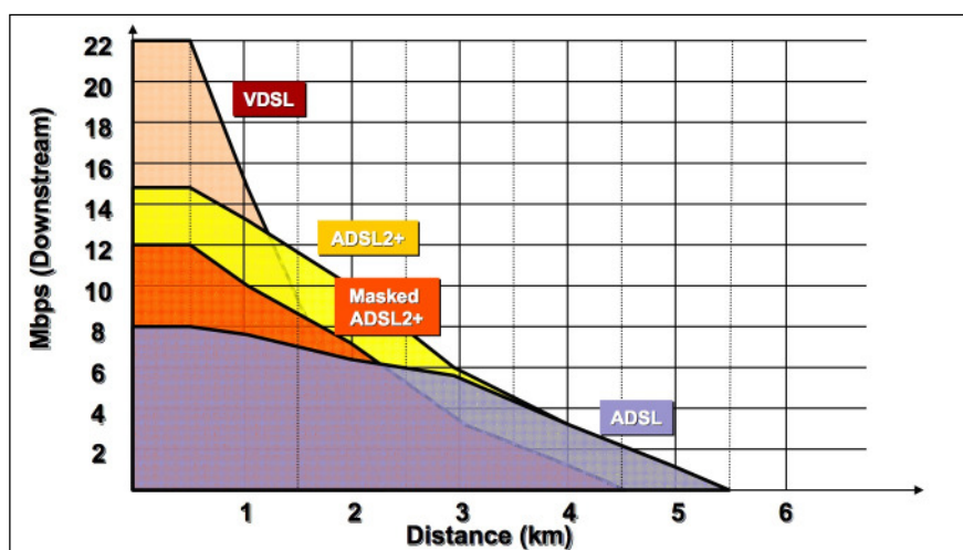
Abbildung 5: Zusammenhang von Leitungslänge und möglicher Zugangsgeschwindigkeit verschiedener xDSL-Technologien Quelle: Ransom 2004.
