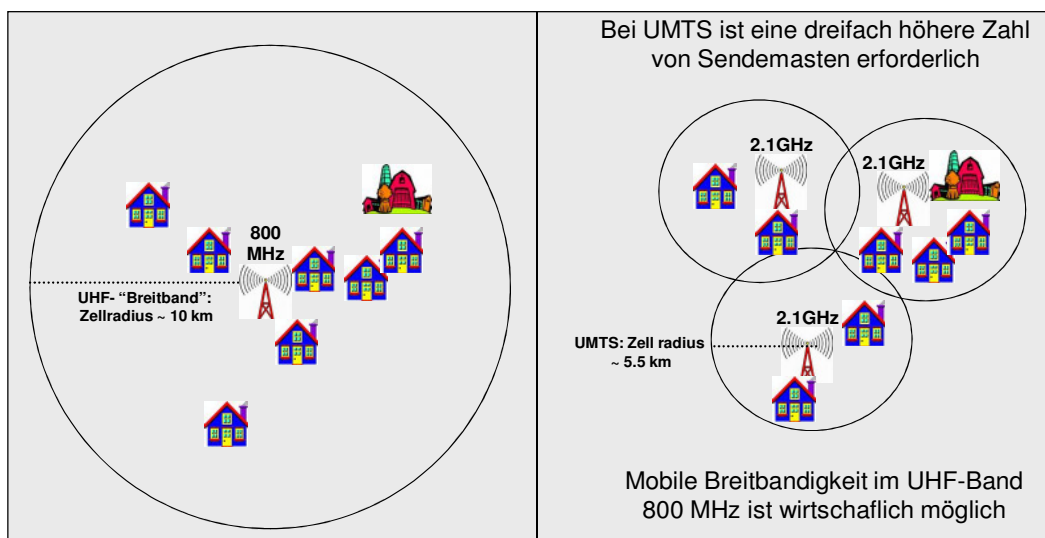
Abbildung 11: Reichweite von Breitband-Mobilfunk bei unterschiedlichen Frequenzen Quelle: Laudan 2008.
